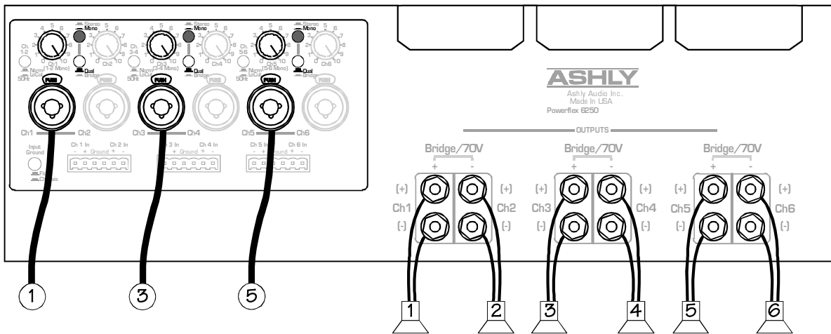
Amplifier Inputs
